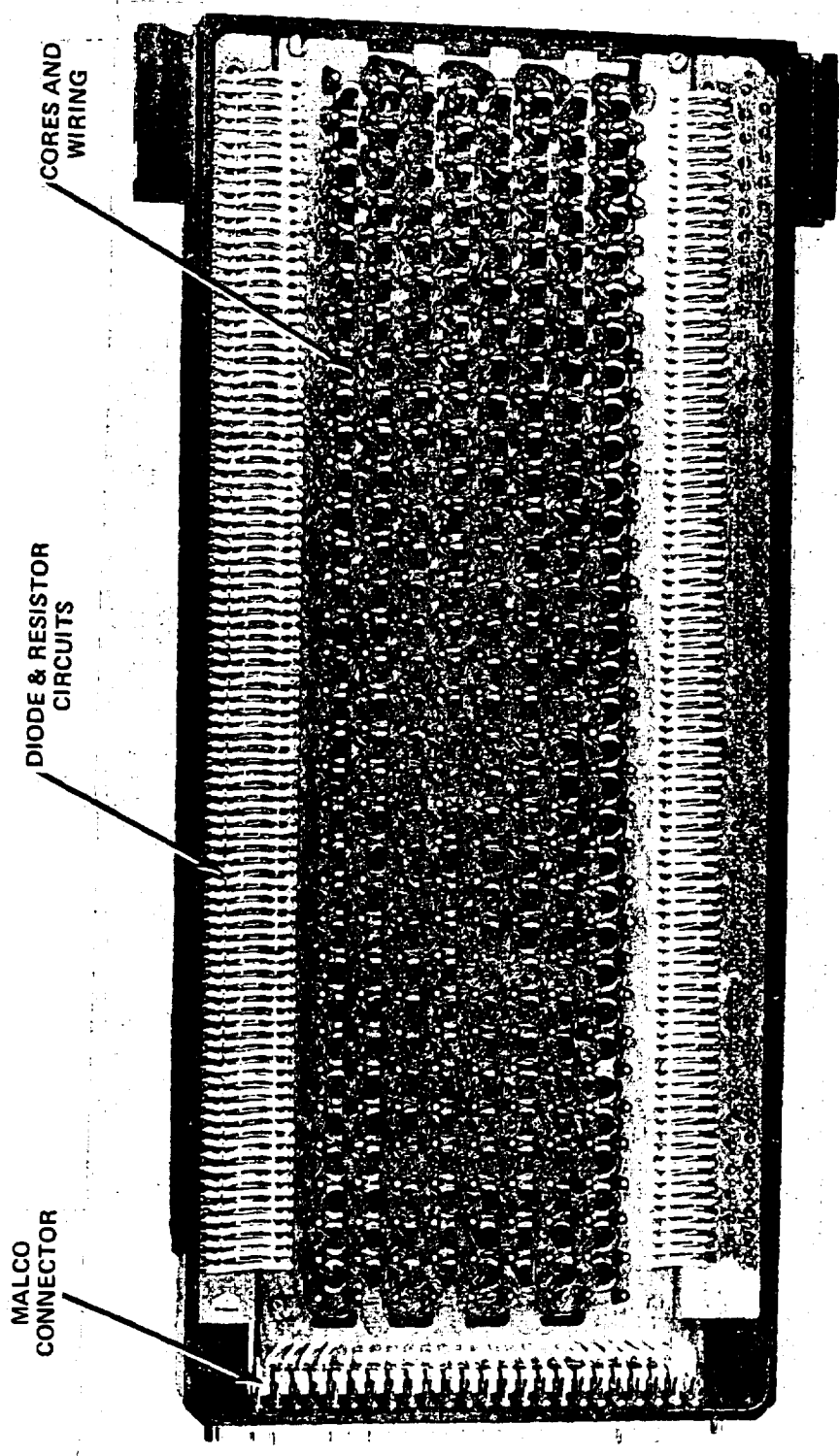
Fig. 3-34 Core Rope Module
