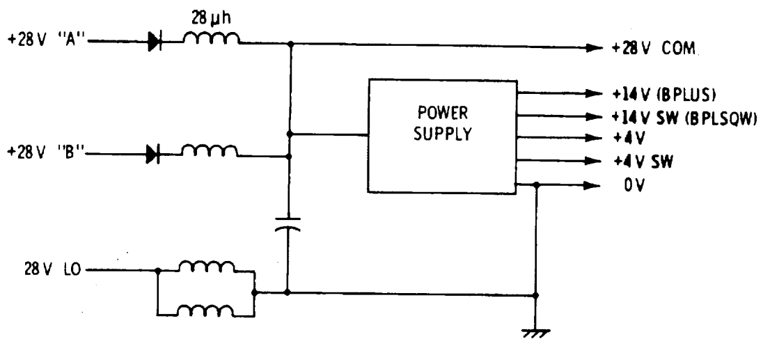
Fig. 6-7 28 Volt DC Input Power
