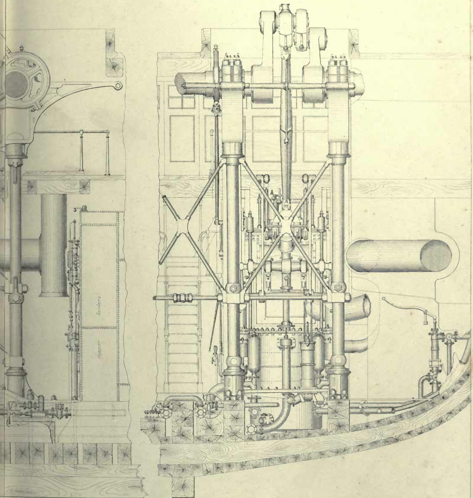
END ELEVATION
