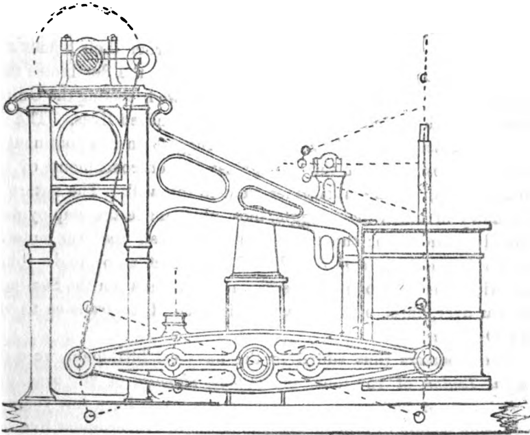
SIDE LEVER ENGINE, U. S. S. MISSISSIPPI.
