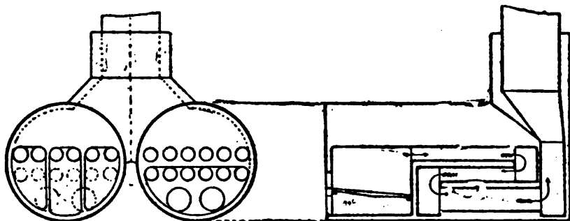
RETURN DROP-FLUE BOILERS, U. S. S. FULTON(3D), 1850.
