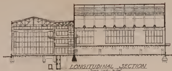
LONGITUDINAL SECTION Scale 1/8" = 1'-0"
