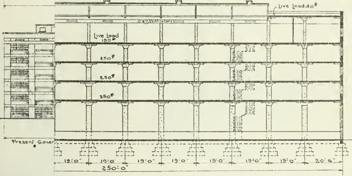
Longitudinal Section —
