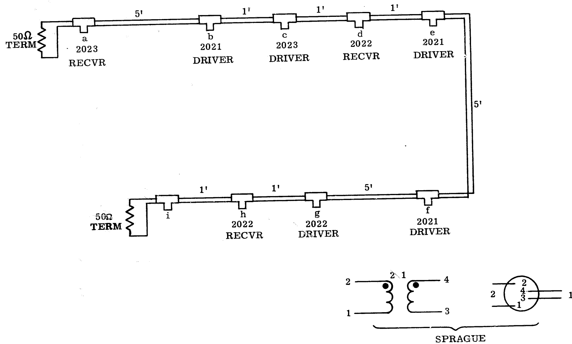
Fig. 3.9 Test layout.
