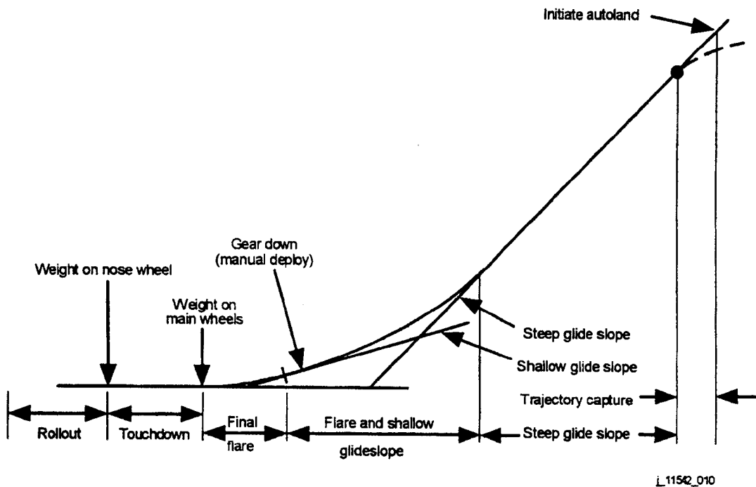
Figure 2-7. A/L longitudinal trajectory
