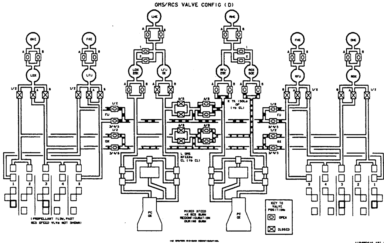
Figure 4-16. OMS/RCS valve configuration (D)
