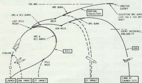
Ascent Trajectory
