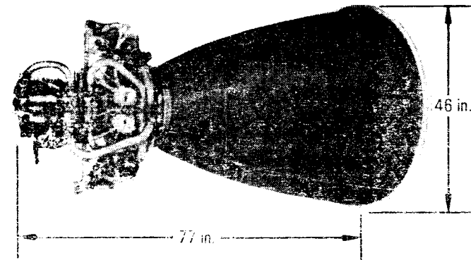
OMS Engine
