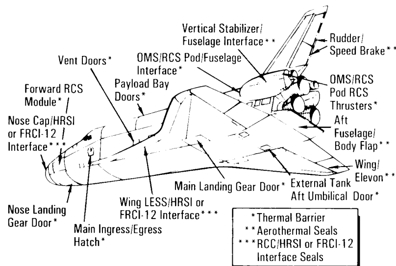
Thermal Barriers
