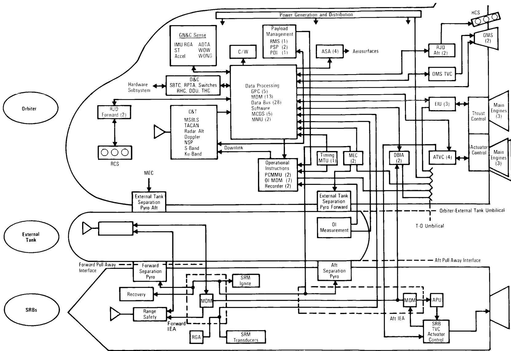
Avionics
