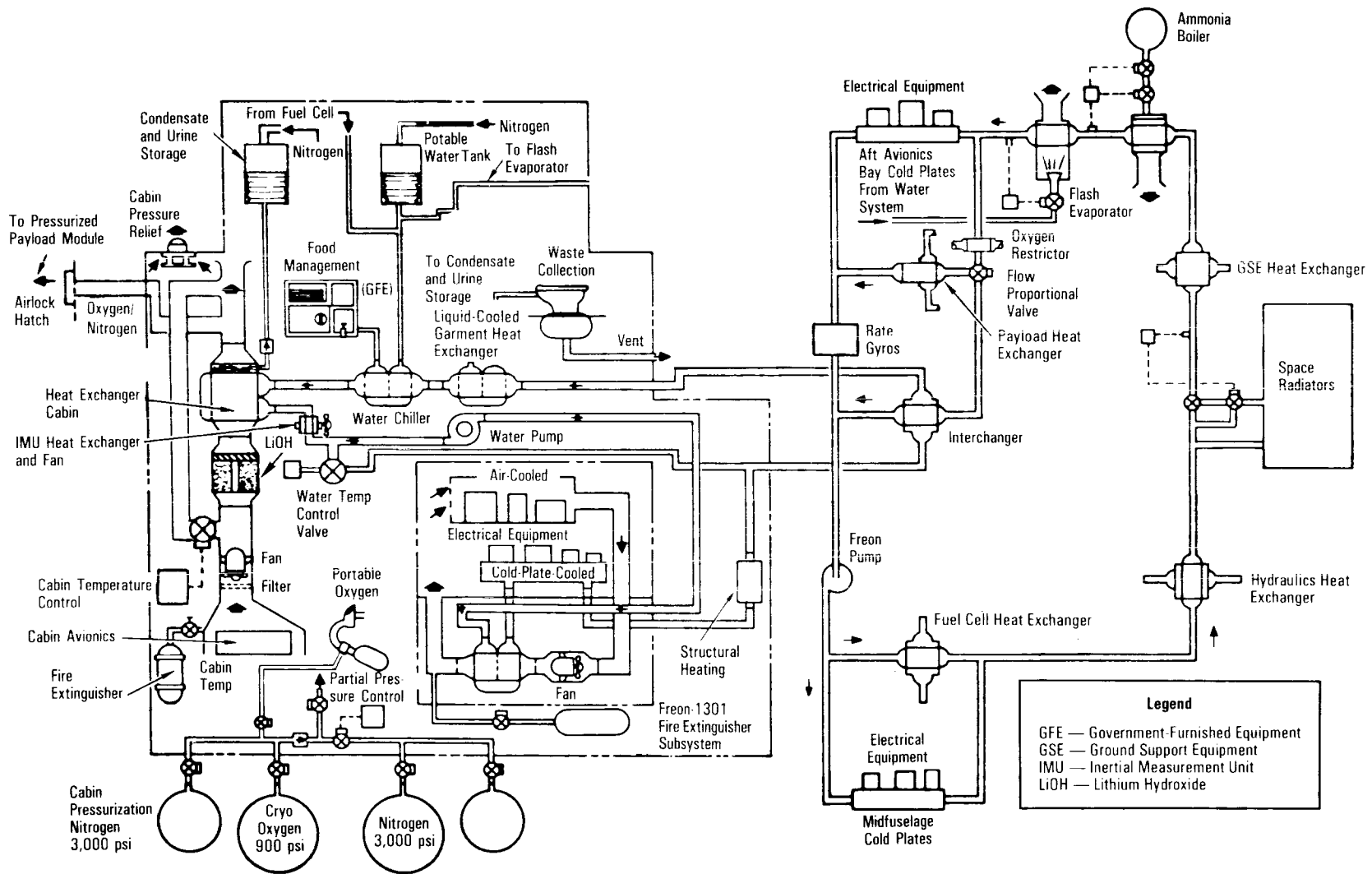
ECLSS Schematic
