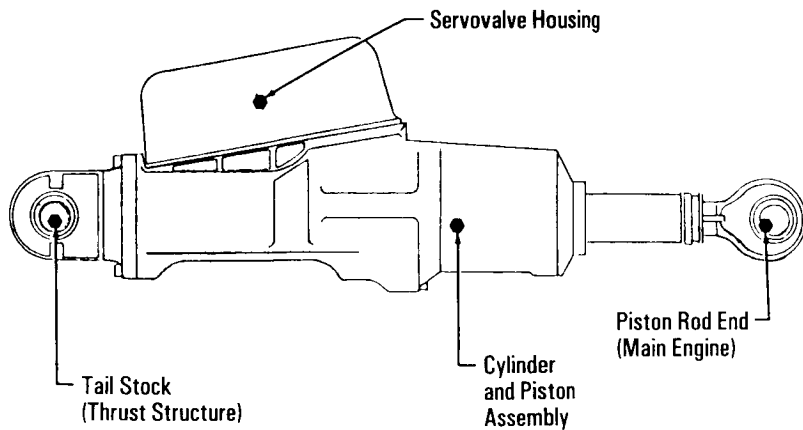
Main Engine Electrohydraulic Servoactuator
