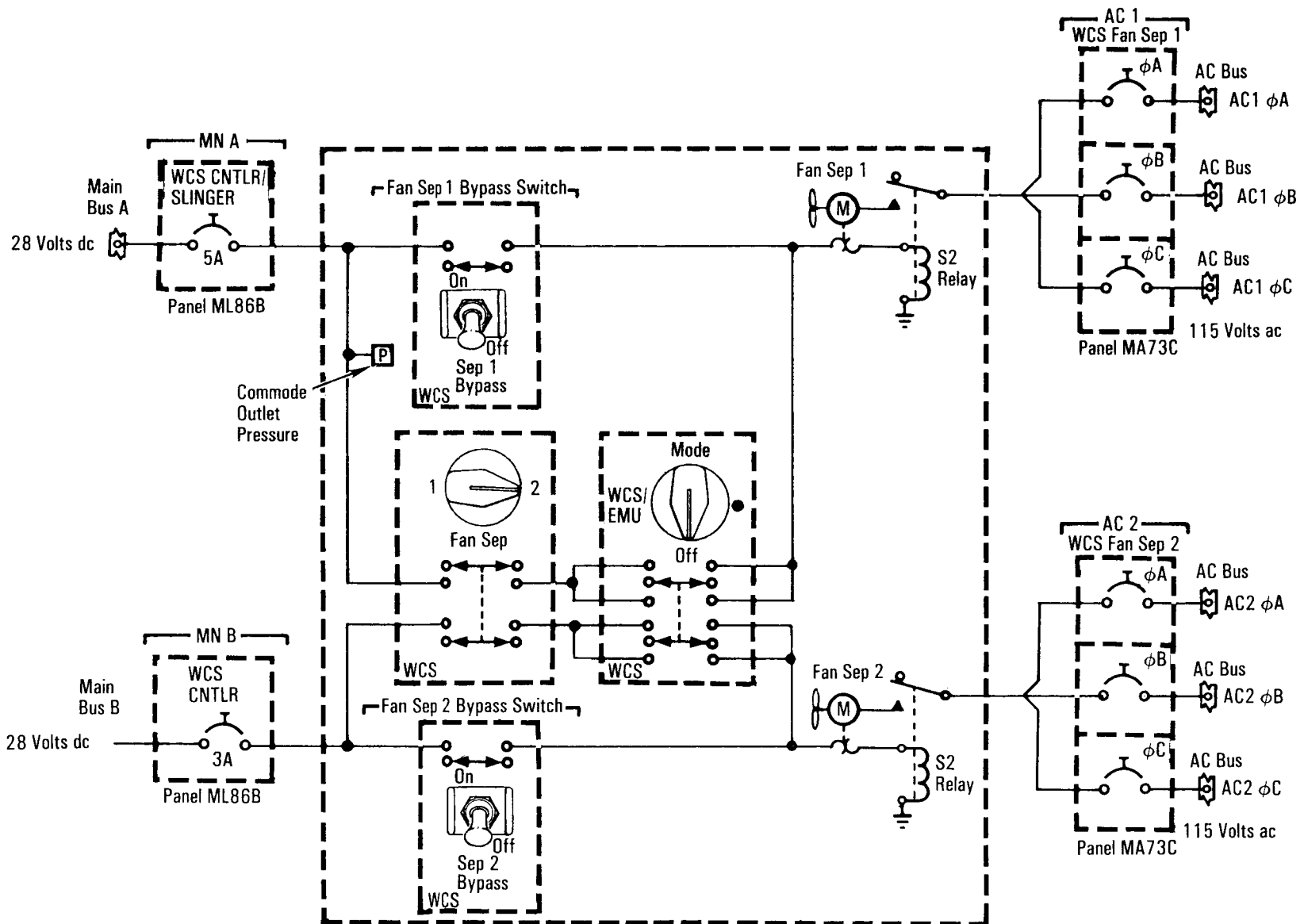
Fan Separator Control
