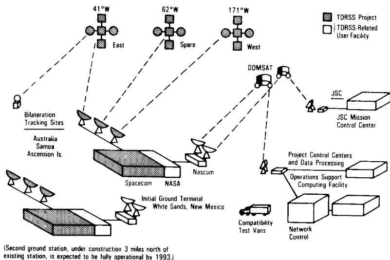
TDRSS Elements
