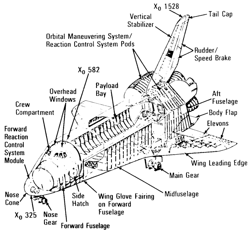
Orbiter
