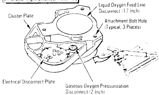
ET Orbiter Right Umbilical Assembly
