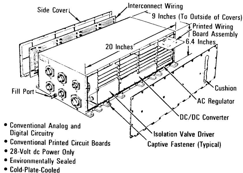
Aerosurface Servoamplifier
