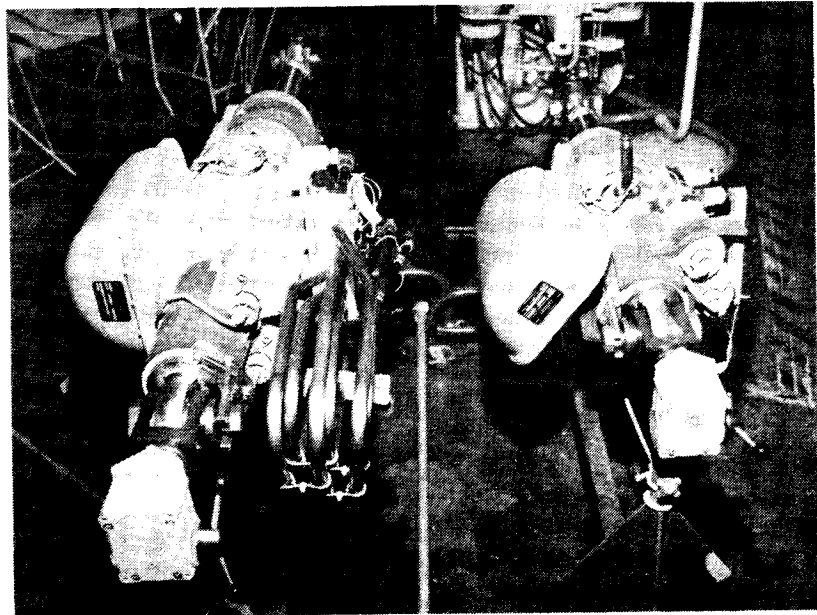
Elevon Actuators
