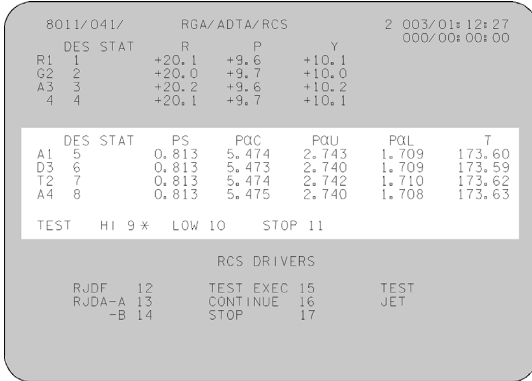
Figure 5-4. RGA/ADTA/RCS (SPEC 41) display
