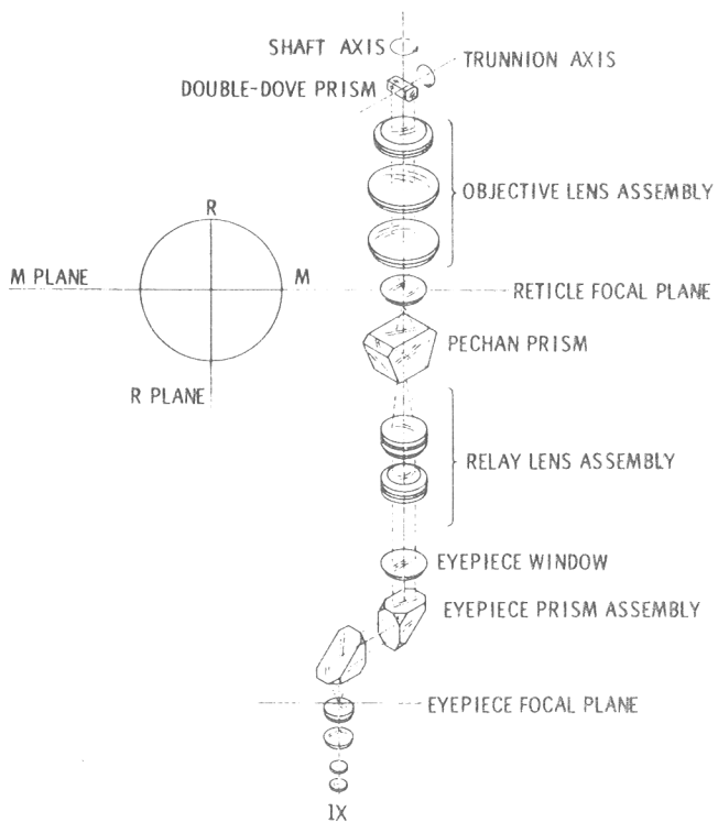
Fig. 3a SCT Optics.
