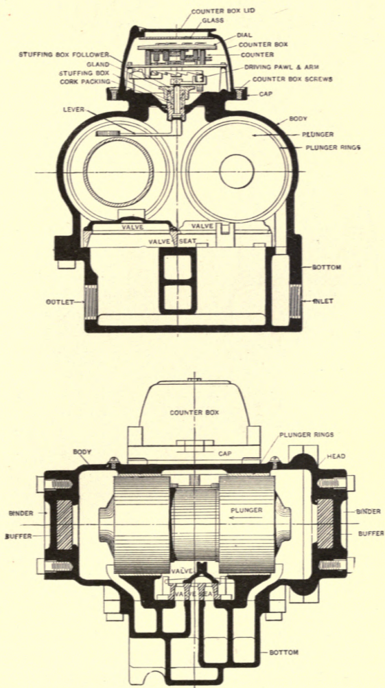
Fig. 78 Duplex Piston Meter
