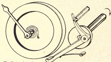
Fig. 200 - Inertia tachometer
