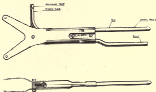
Fig. 211. Pitot Tube
